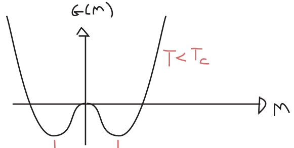
dois mínimos com magnetizações opostas
